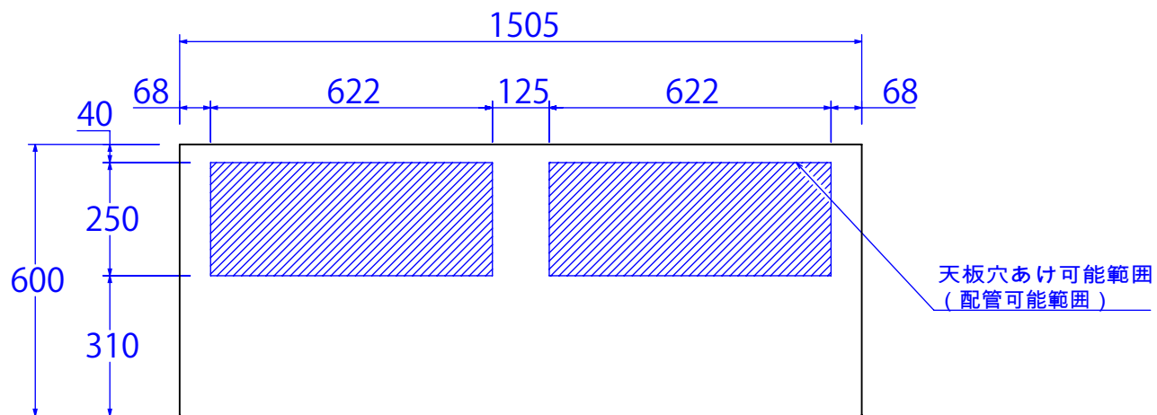
上面図
