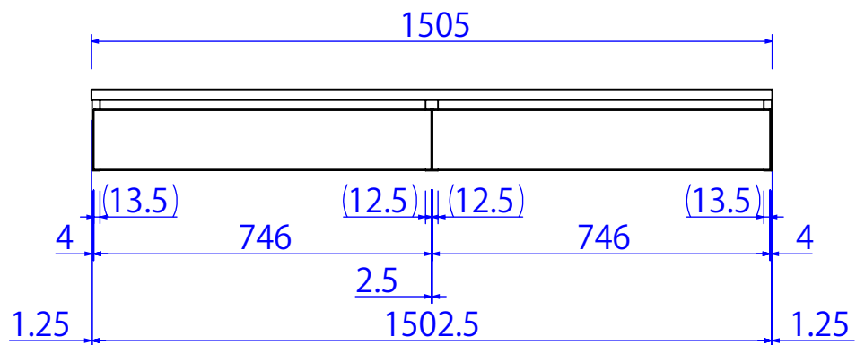
正面図
